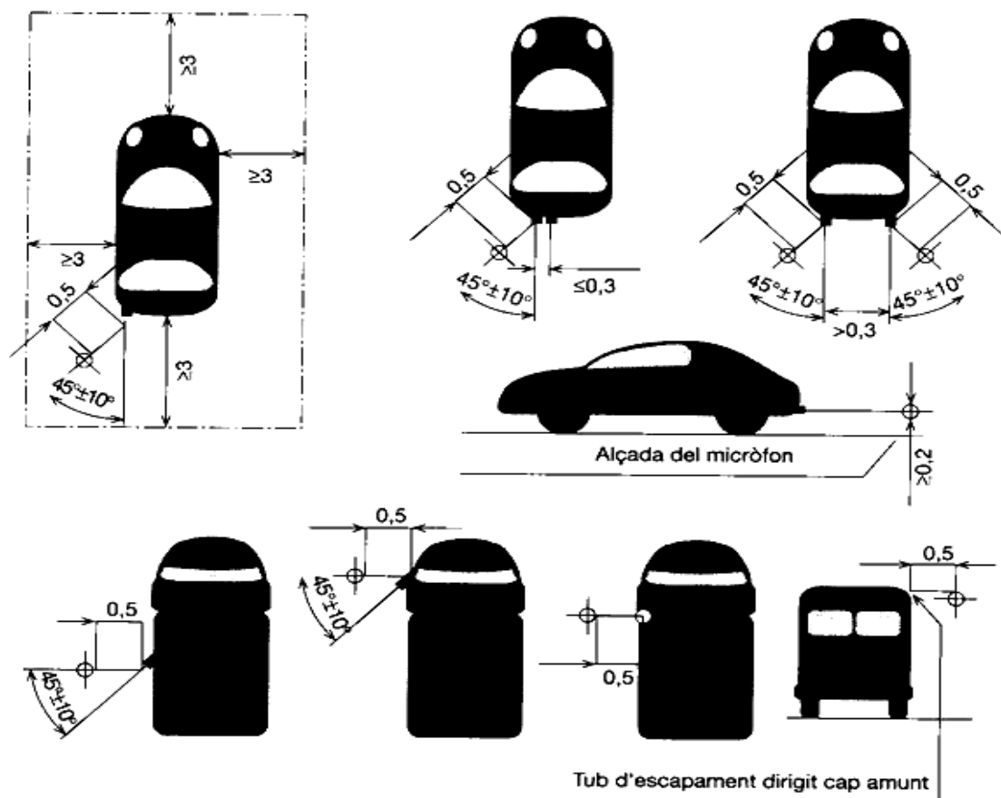
Figura 2. Posición del instrumento de medida en vehículos automóviles
